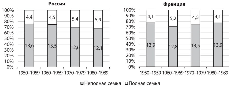
Рисунок 4. Среднее время (значения в годах указаны в столбцах) и доли периода детства до 18 лет, проведенные детьми в полных и неполных семьях среди рожденных в полных семьях (А) и в неполных семьях (Б), поколения детей по году их рождения, Россия и Франция. Источник: расчеты авторов.
